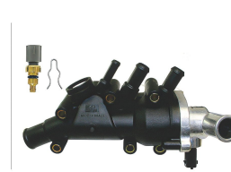
KIT CAVALETE DE DISTRIBUIÇÃO DE ÁGUA CARÇAÇA/ SENSOR/ VÁLVULA
