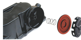
KIT DE REPARO DA TAMPA
