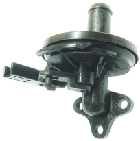
VÁLVULA DO AR QUENTE
