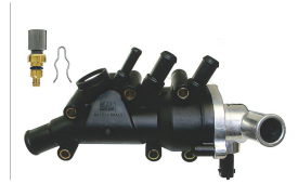
KIT CAVALETE DE DISTRIBUIÇÃO DE ÁGUA CARÇAÇA/ SENSOR/ VÁLVULA
