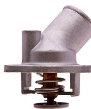
VÁLVULA TERMOSTÁTICA
