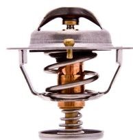
VÁLVULA TERMOSTÁTICA
