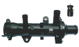
KIT CAVALETE DE DISTRIBUIÇÃO DE ÁGUA CARÇAÇA/ TAMPA/ VÁLVULA
